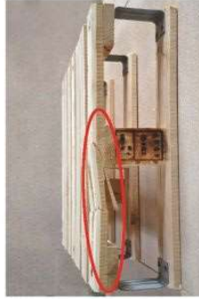
Deska góra lub dolna z pęknięciem poprzecznym
