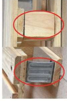
Wspornik metalowy bez logotypu, drewniany wspornik bez oznaczeń lub deski o grubości poniżej 20 mm
